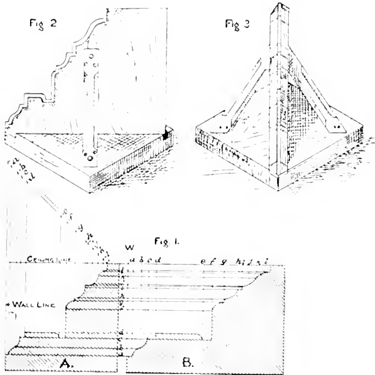
NO. 17.—MITRE-MOULD.
